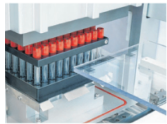
Die Montagelinie BCT-200 stellt Blutentnahmeröhrchen her und verpackt diese. In die Röhrchen werden Additive dosiert, anschließend folgt das Verschließen unter Vakuum.
